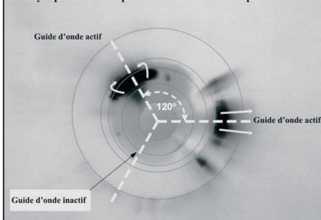
Analyse photo de la coque inférieure du TR3A "Sportster" en vol
