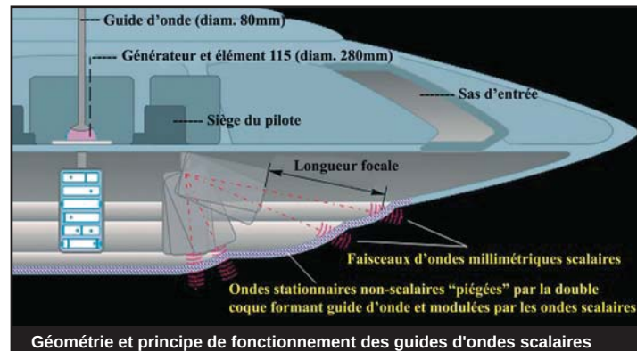
Géométrie et principe de fonctionnement des guides d'ondes scalaires
