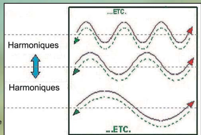
Le potentiel scalaire
